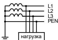
Схема TN-C
