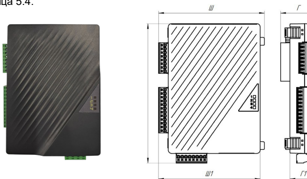
Рисунок 5.7 – Модуль INMX-Ecard
