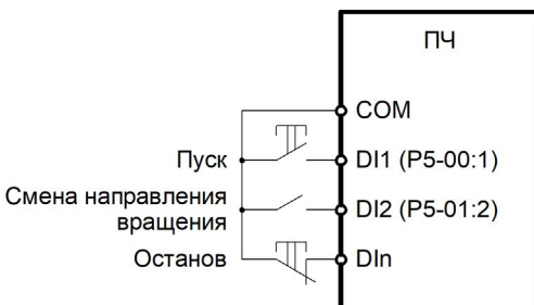
Рисунок 6.12– Схема трехпроводного подключения 2
