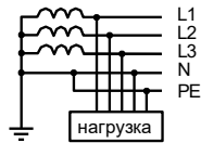
Схема TN-C-S
